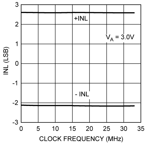
3V INL vs. f_{SCLK}
